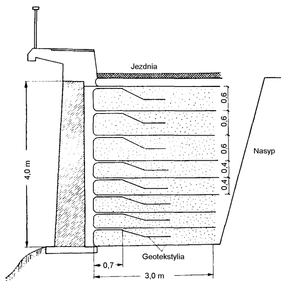
Rys. 4.1. Wzmocnienie ściany oporowej za pomocą zbrojenia gruntu geotekstylami
