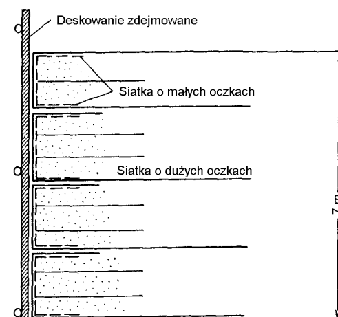
Rys. 4.2. Ściana z gruntu zbrojonego geotekstylami siatkowymi
