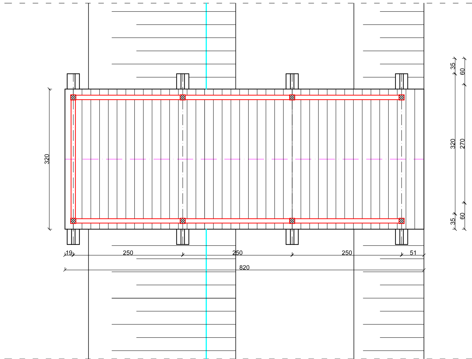
Pomost widokowy skala 1:50 Rzut z góry
