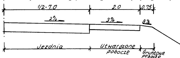
Rys. nr 1. Przykład utwardzonego pobocza o grubości mniejszej niż grubość jezdni
