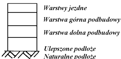
Rys. nr 3. Konstrukcja nawierzchni utwardzonego pobocza
