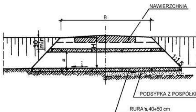
Rys. nr 1. Przekrój podłużny przepustu z rury polietylenowej średnicy 40÷50 cm pod zjazdem
