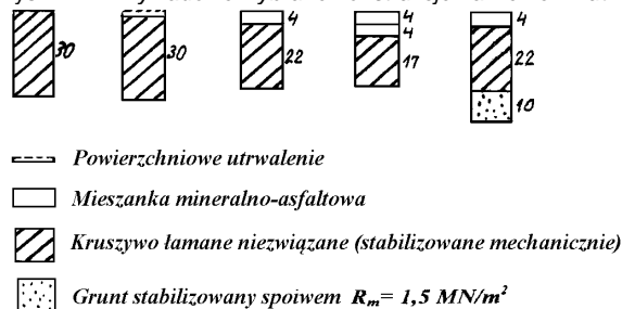
Rys. nr 4. Przykładowe wybrane konstrukcje nawierzchni utwardzonego pobocza z kruszywa łamanego niezwiązanego
