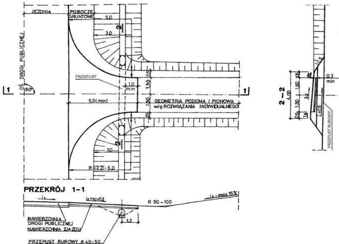
Rys. nr 2. Przykładowe rozwiązanie sytuacyjne zjazdu indywidualnego z przepustem
