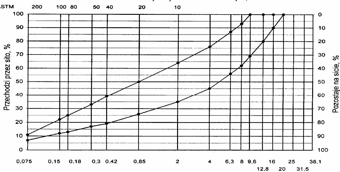
Wymiary oczek sit kwadratowych, mm
