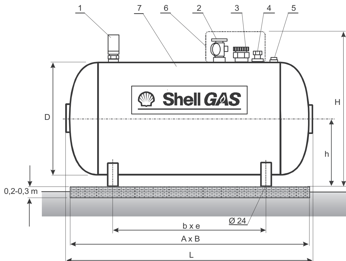
Rys. 3. Naziemny zbiornik magazynowy LPG
