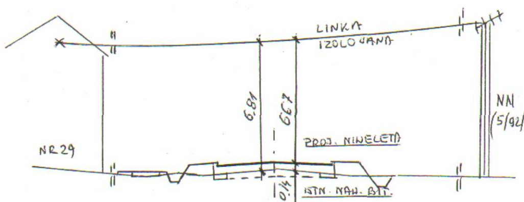
Profil na skrzyżowaniu linii NN w km 4+762
