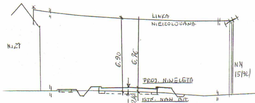
Profil na skrzyżowaniu linii NN w km 4+738
