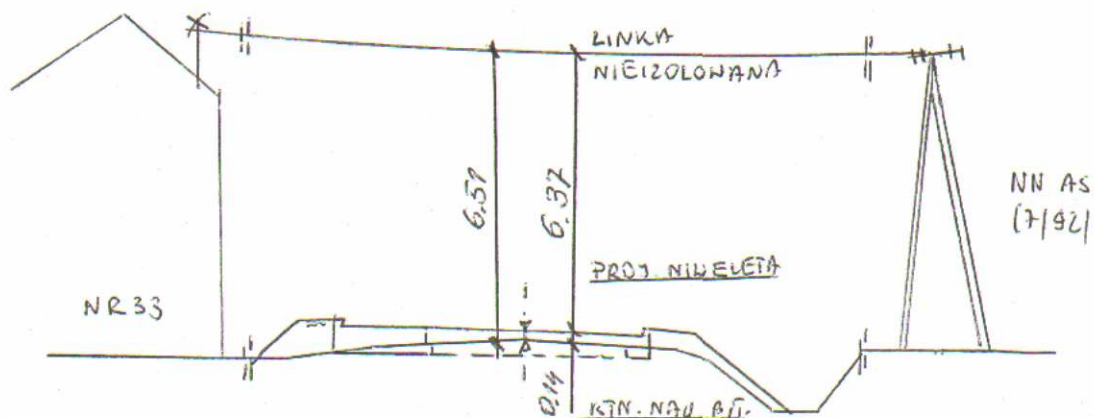
Profil na skrzyżowaniu linii NN w km 4+795
