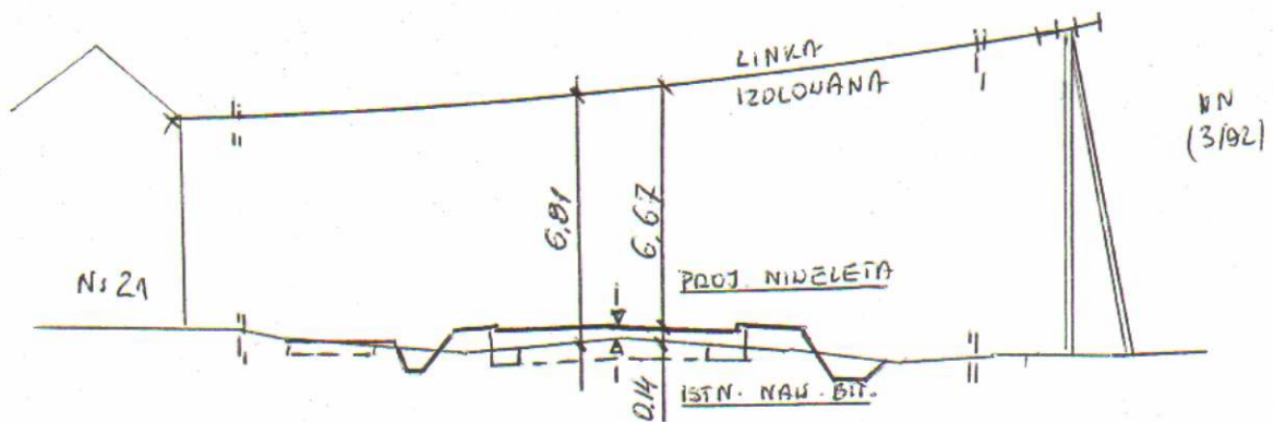
Profil na skrzyżowaniu linii NN w km 4+701.50
