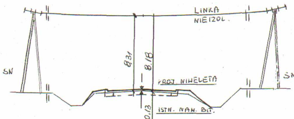
Profil na skrzyżowaniu linii NN w km 4+568
