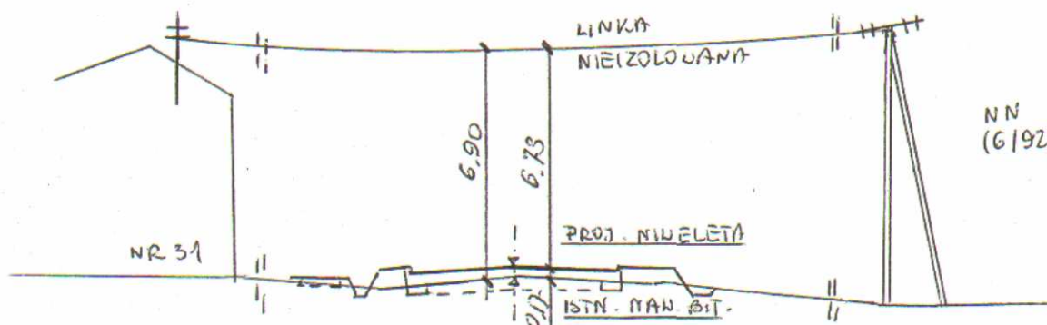
Profil na skrzyżowaniu linii NN w km 4+795
