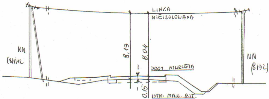
Profil na skrzyżowaniu linii NN w km 4+898
