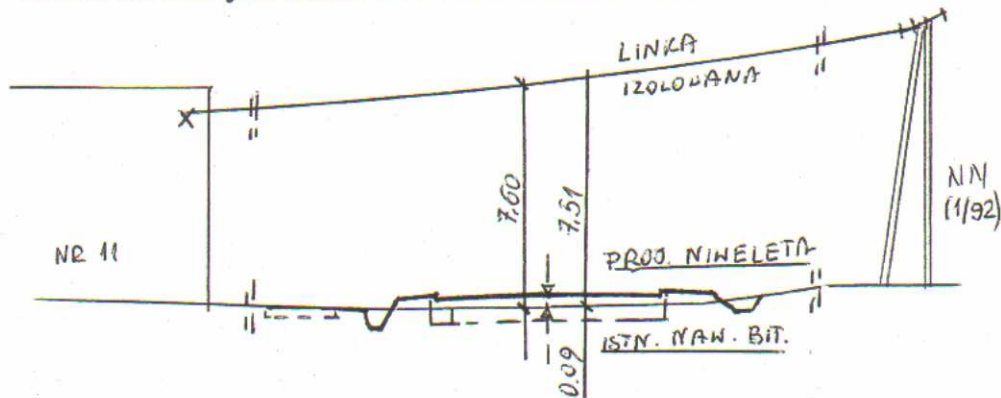
Profil na skrzyżowaniu linii NN w km 4+601
