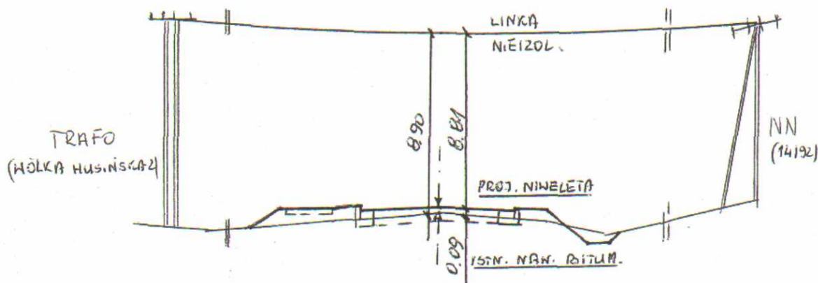
Profil na skrzyżowaniu linii NN w km 4+594
