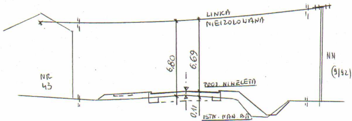
Profil na skrzyżowaniu linii NN w km 4+933
