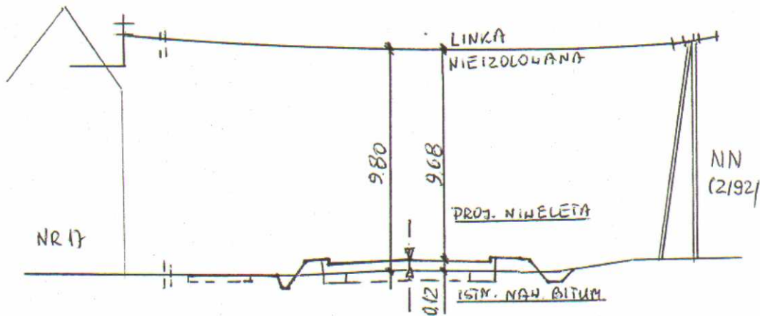
Profil na skrzyżowaniu linii NN w km 4+666.80
