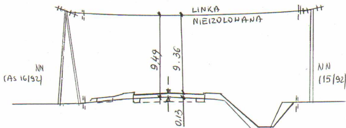
Profil na skrzyżowaniu linii NN w km 4+991.50
