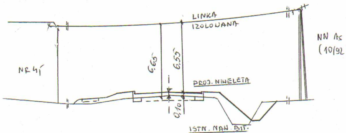
Profil na skrzyżowaniu linii NN w km 4+943.50
