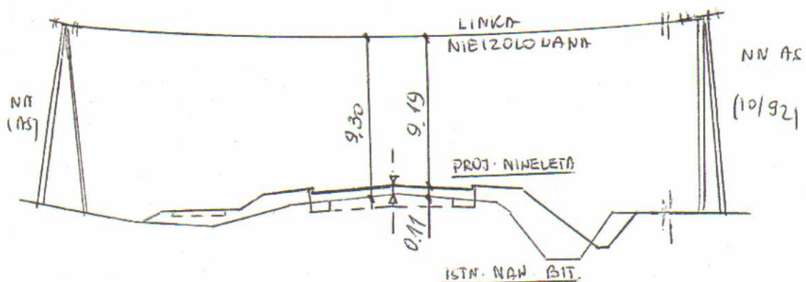
Profil na skrzyżowaniu linii NN w km 4+943.50
