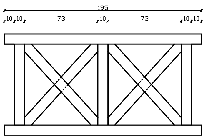
SEGMENT BARIERKI 10D
